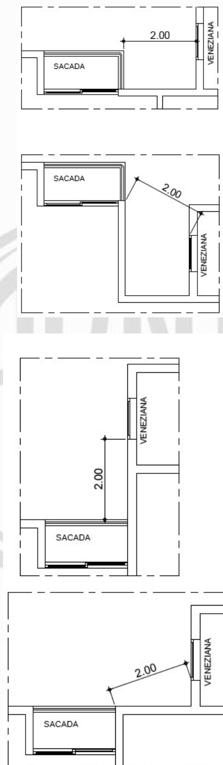
Figura 9 – Distâncias mínimas entre as venezianas da escada EP e outro tipo de abertura em planos distintos
