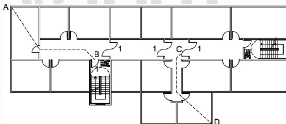
c) Exemplo 03 – Exemplo de compartimentação horizontal composto áreas de refúgio adequadas ao abandono horizontal progressivo
