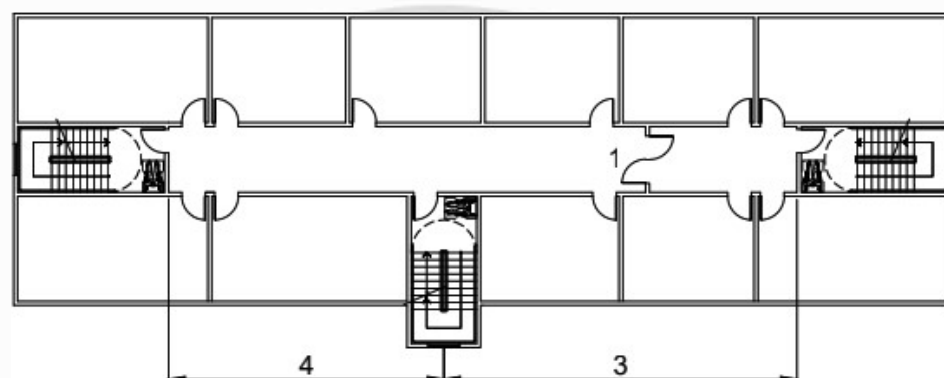
b) Exemplo 02 – Corredor com três saídas verticais
