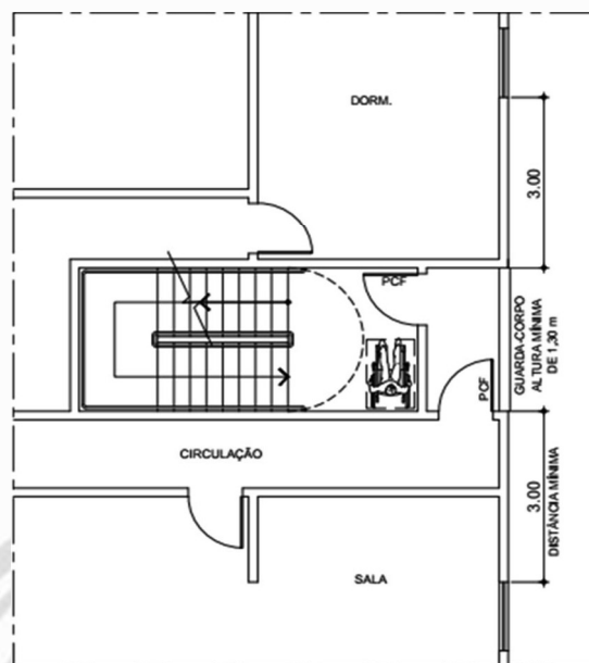
Figura 11 – Escada protegida com ventilação em seu acesso
