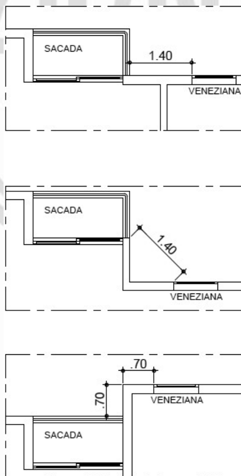
Figura 8 – Distâncias mínimas entre as venezianas da escada EP e outro tipo de abertura no mesmo plano
