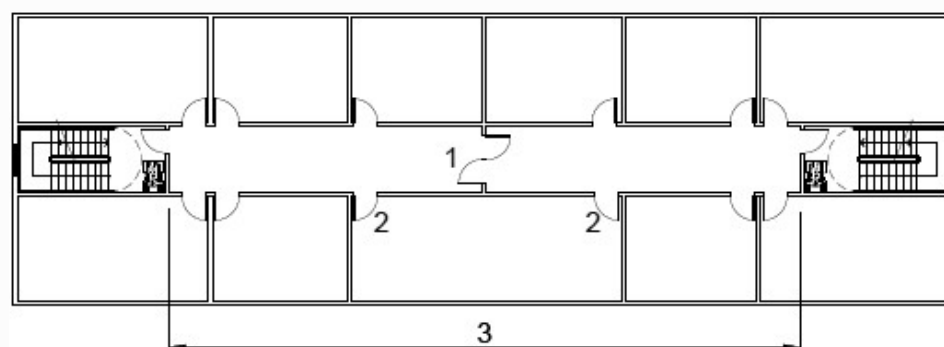
a) Exemplo 01 – Corredor com duas saídas verticais
