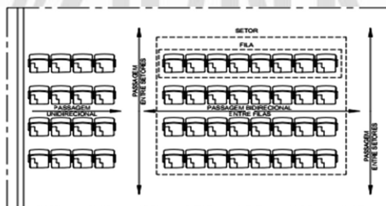
Figura 6 – Setores e fileiras de assentos fixos
