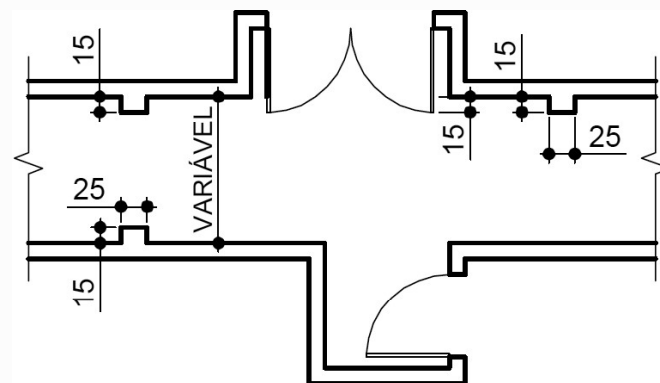
Figura 4 – Medidas da largura em saídas horizontais e reduções admissíveis
