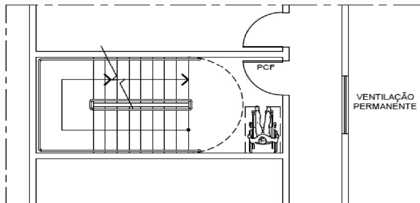
Figura 10 – Exemplo de escada protegida com ventilação em seu acesso
