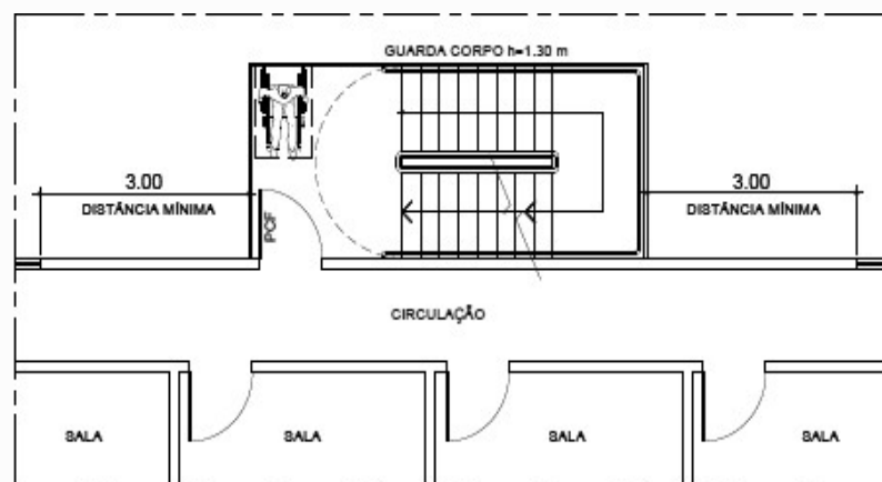
Figura 12 – Escada externa
