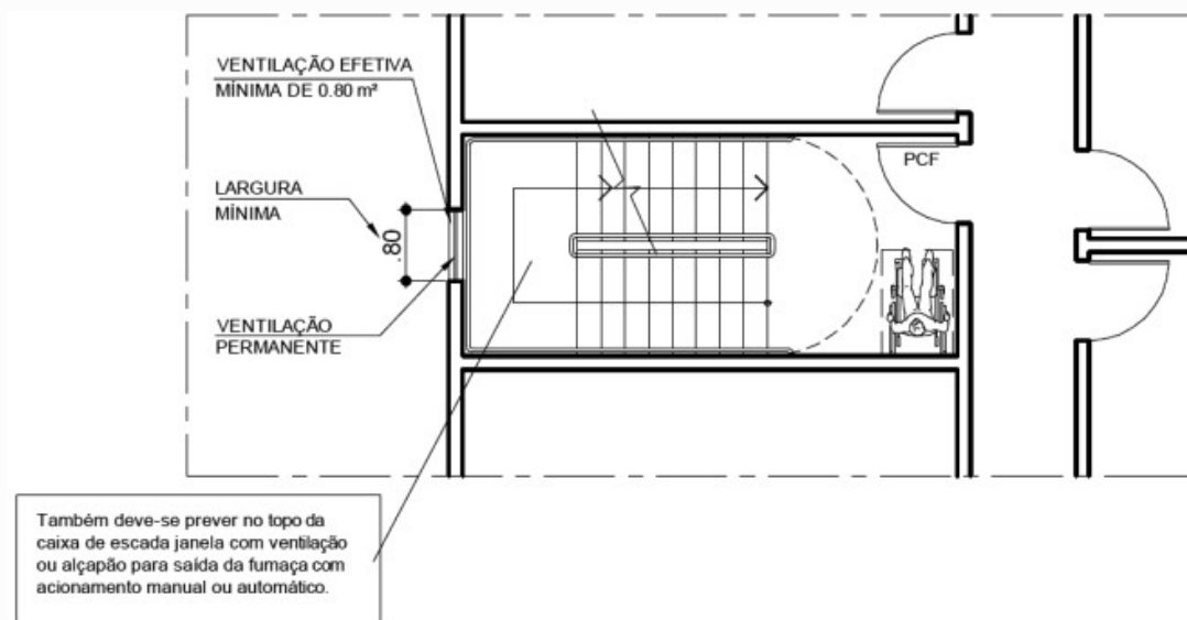
Figura 7 – Exemplo de escada protegida
